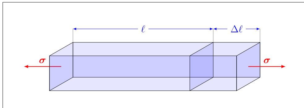
Abbildung 1.12: Lineare Verformung eines Stabes durch die Zugspannung \sigma .
