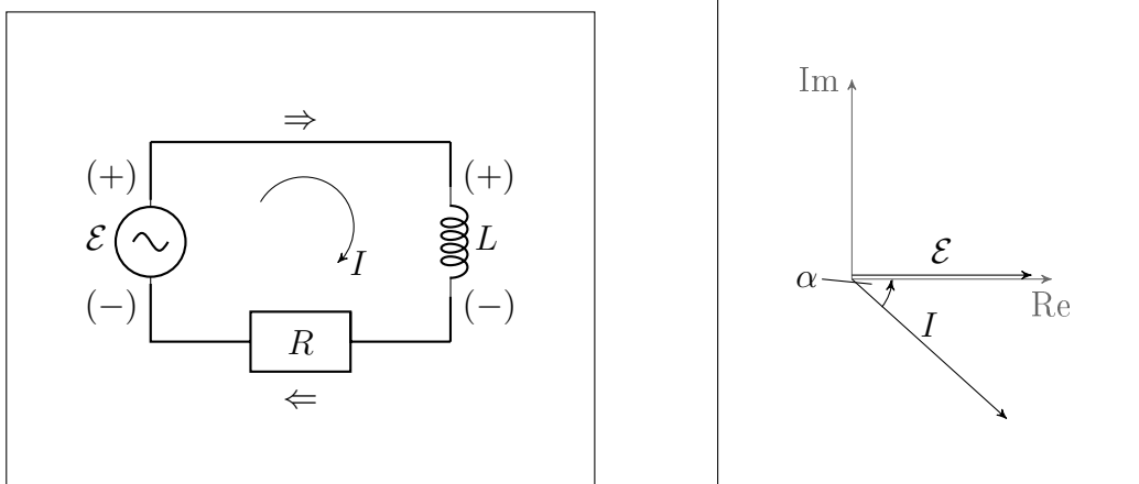
(a) Einfacher RL -Stromkreis. Eine momentane Stromrichtung (Polarität von \mathcal{E} in Klammern) ist eingezeichnet.
