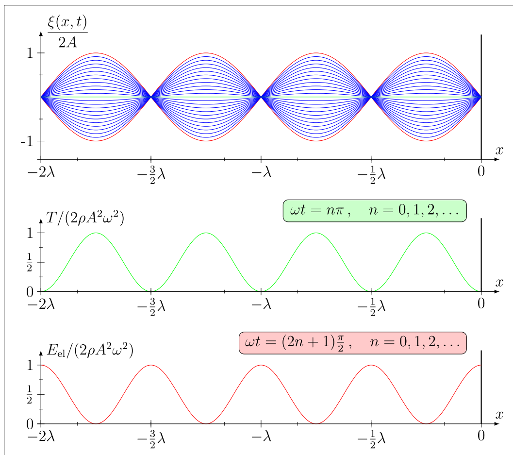
Abbildung 1.31: Verteilung der kinetische Energie T und der elastischen Energie E_{\text{el}} bei einer stehende Welle für die Reflexion am harten Medium ( \alpha \gg 1 ).
