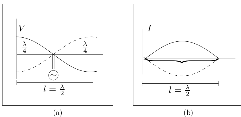
Abbildung 10.10: (a) Stehende Spannungswelle auf einem \lambda/2 Dipol zu einem Zeitpunkt, an dem die Spannungsdifferenz zwischen den Dipolenden maximal ist. (b) Stehende Stromverteilung eines \lambda/2 Dipols.
