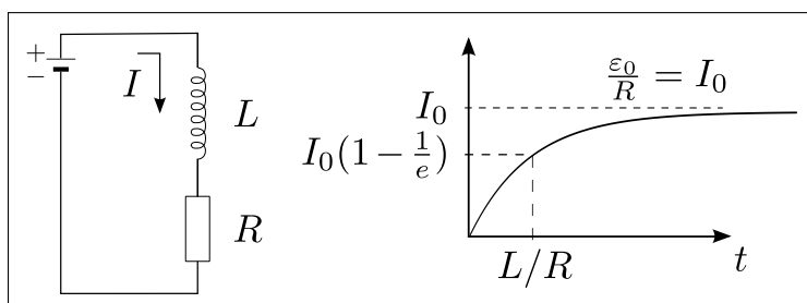
(b) Zeitverhalten nach Schliessen des Schaltkreises.
