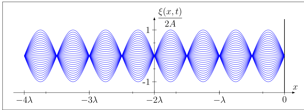
Abbildung 1.29: Stehende Welle bei Reflexion am harten Medium ( \alpha \gg 1 ).
