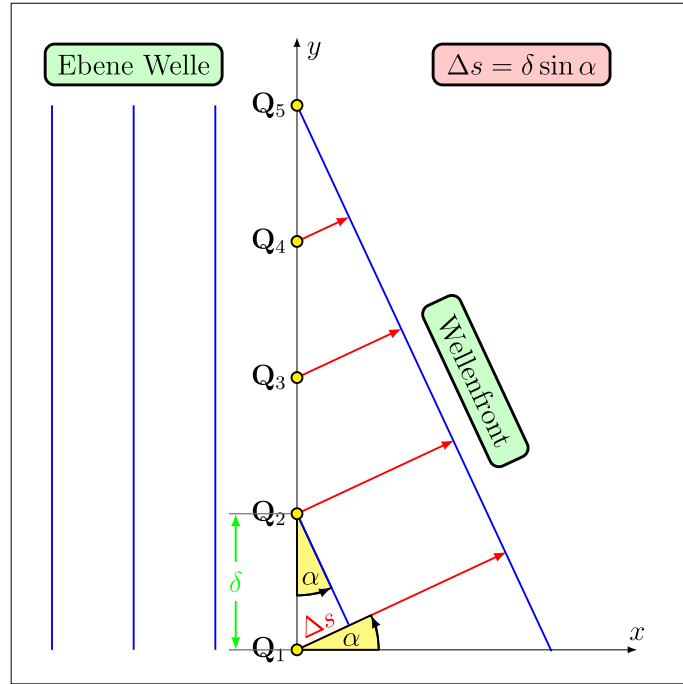
Abbildung 1.39: Überlagerung der von N Quellen auslaufenden Kugelwellen in Richtung des Winkels \alpha .
