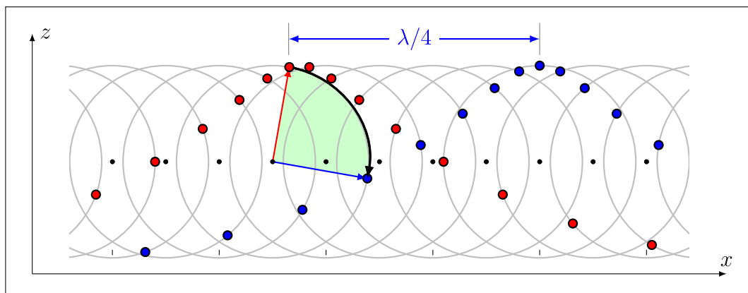
Abbildung 1.51: Nach rechts wandernde Wasserwelle zu den Zeiten t = 0 und t = T/4 .
