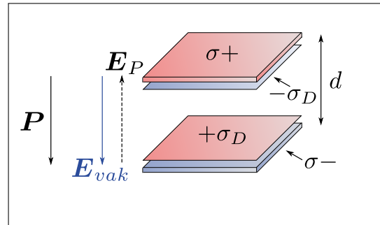
(c) Die Ausrichtung des elementaren Dipole erzeugt effektiv eine Flächenladungsdichte \sigma_D , die die Flächenladungsdichte auf den Kondensatorplatten schwächt.
