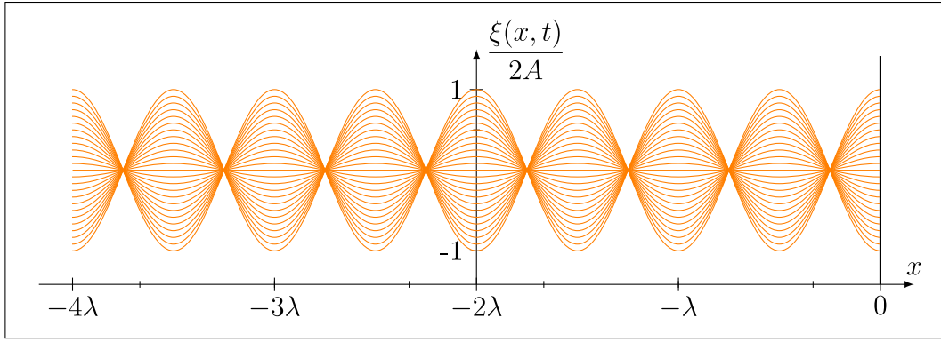
Abbildung 1.30: Stehende Welle bei Reflexion am weichen Medium ( \alpha = 0 ).
