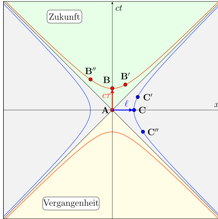
Abbildung 5.8: Lichtkegel und Kausalität. Die Punkte B , B' und B'' können von A aus erreicht werden und weisen alle dieselbe Eigenzeit c\Delta\tau = \sqrt{\Delta s^2} aus. Die Punkte C , C' und C'' haben alle dasselbe raumartige Raumzeit-Intervall \Delta\ell = \sqrt{-\Delta s^2} und können von A aus nicht erreicht werden.
