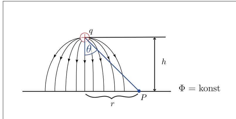
(a) Eine Ladung im Abstand h über einer unendlich ausgedehnten Leiterplatte induziert eine Oberflächenladungsdichte \sigma_{\text{ind}} , sodass \int \sigma_{\text{ind}} da = -q ist.
