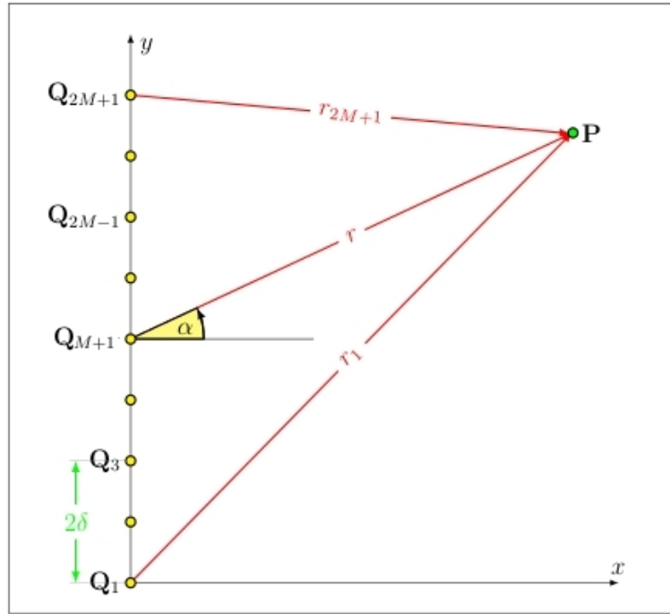
Abbildung 1.40: Zur Berechnung der Interferenz im Punkte P .
