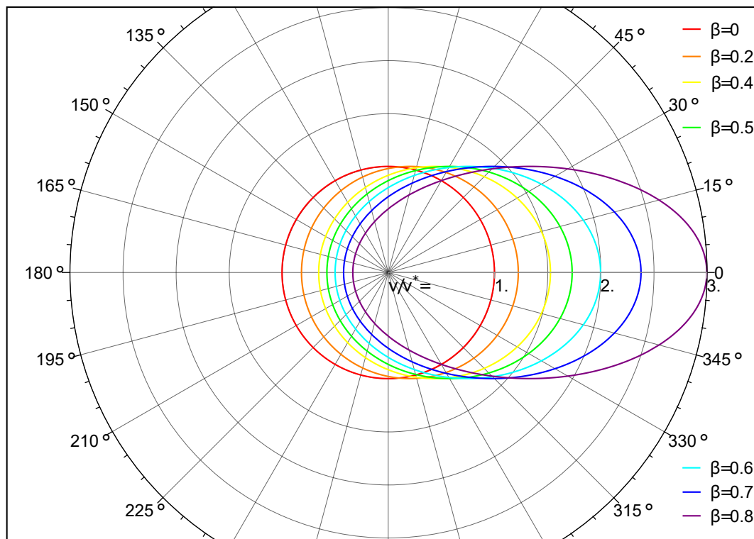
Abbildung 5.14: Relativistischer Dopplereffekt. Polardiagramm des Frequenzverhältnisses \nu/\nu^* in Funktion des Polarwinkels \vartheta im Laborsystem für verschiedene Geschwindigkeiten \beta . Für \beta = 0 ergibt sich der Kreis mit Radius 1.
