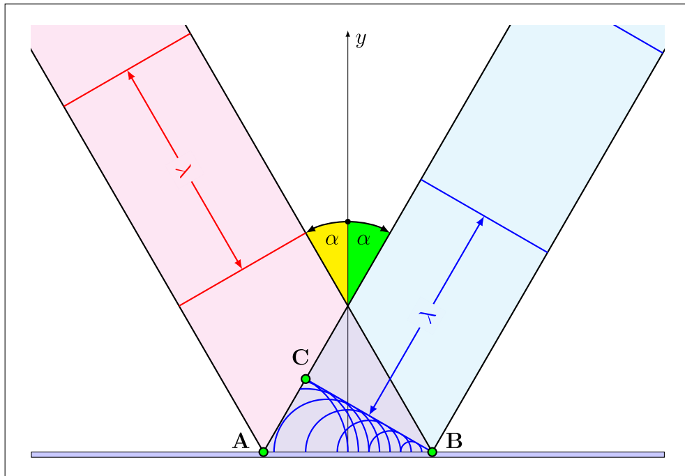
Abbildung 1.43: Huygens'sches Prinzip und Reflexionsgesetz.
