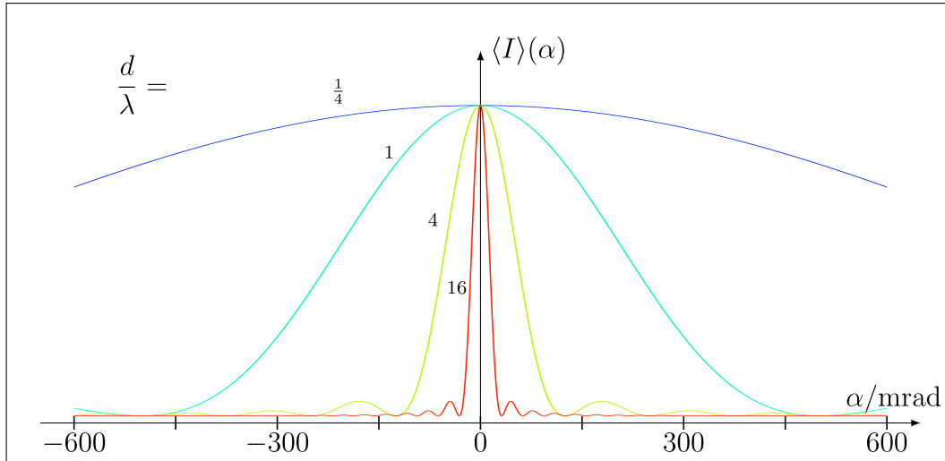
Abbildung 1.42: Beugung am Spalt.
