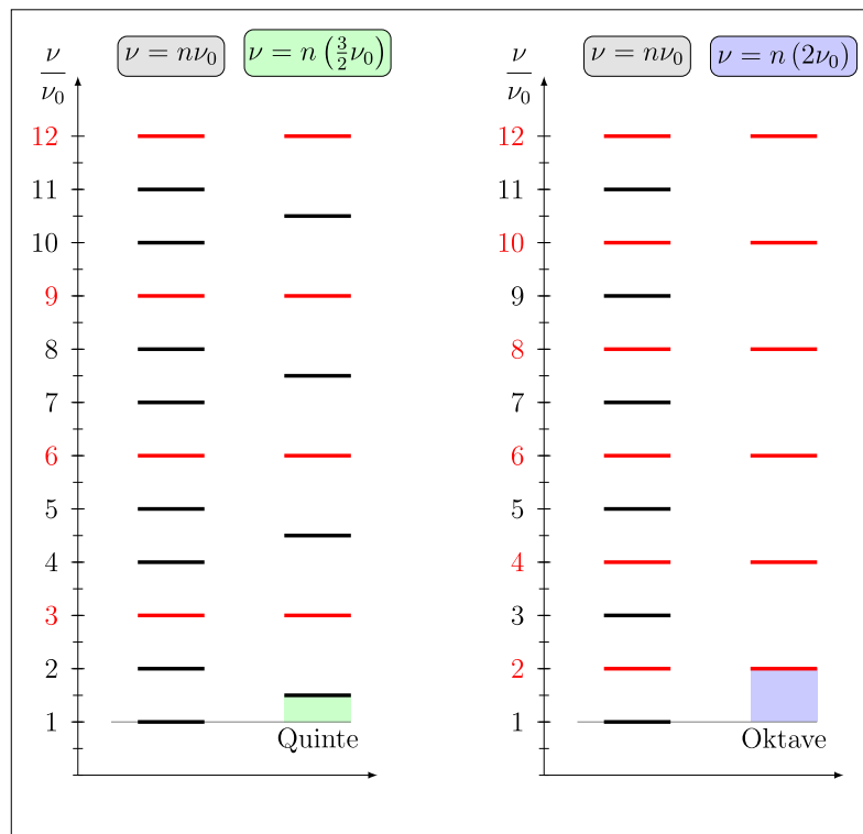
Abbildung 1.36: Die Tonintervalle Quinte und Oktave und gemeinsame Obertöne.
