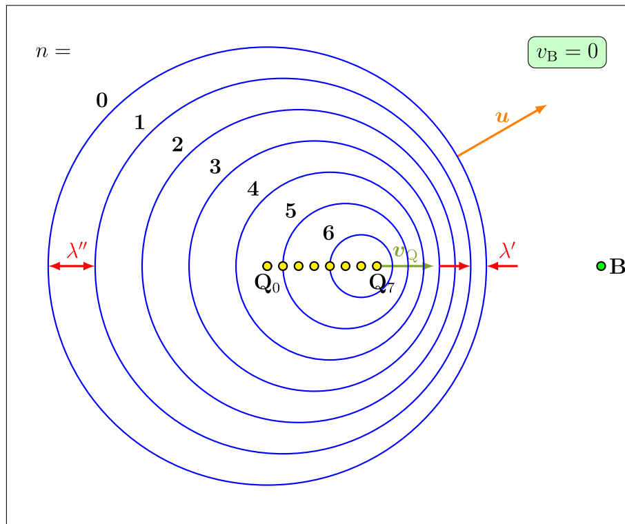
Abbildung 1.56: Dopplereffekt: Bewegte Quelle, ruhender Beobachter.
