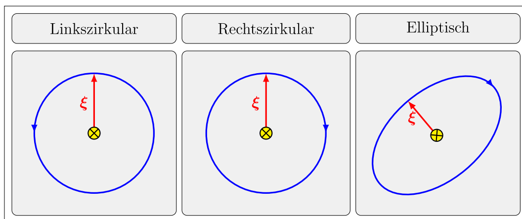
Abbildung 1.18: Zirkulare und elliptische Polarisation.
