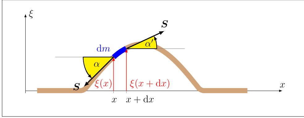
Abbildung 1.10: Auf das Massenelement dm eines Seils wirkende Kräfte.
