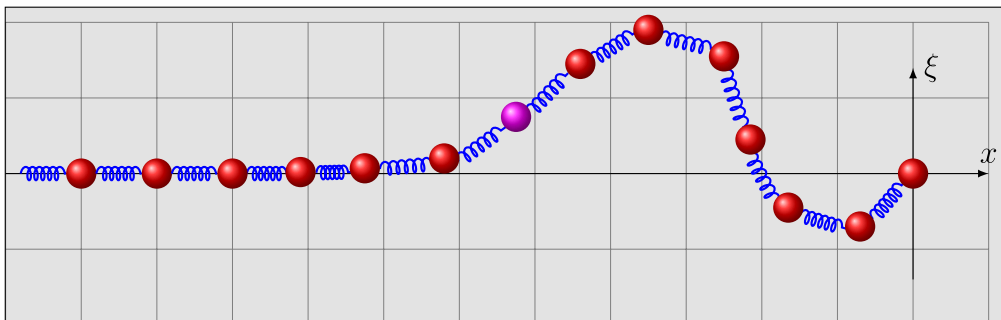
Abbildung 1.4: Transversale Wellen im Masse-Feder-System.
