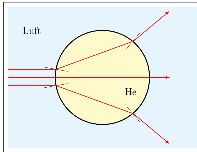
Abbildung 1.47: Defokussierende akustische Linse.
