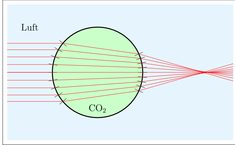
Abbildung 1.48: Fokussierende akustische Linse.
