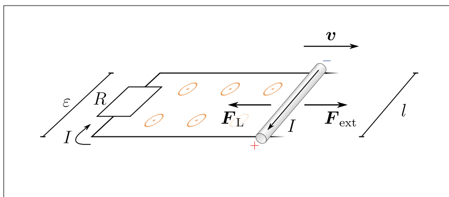
Abbildung 8.6: Ein Stromkreis mit einem bewegten Leiter, an dem eine externe Kraft \mathbf{F}_{\text{ext}} wirkt.
