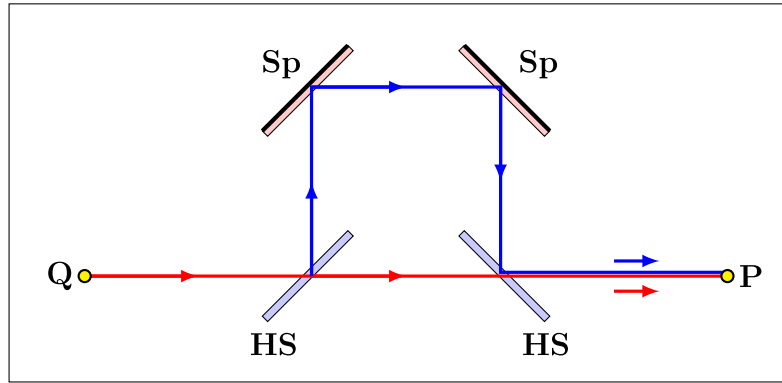
Abbildung 1.23: Aufteilung der von einer Quelle Q erzeugten Welle durch halbdurchlässige Spiegel HS und anschliessende Interferenz im Punkt P . Sp sind nichtdurchlässige Spiegel.
