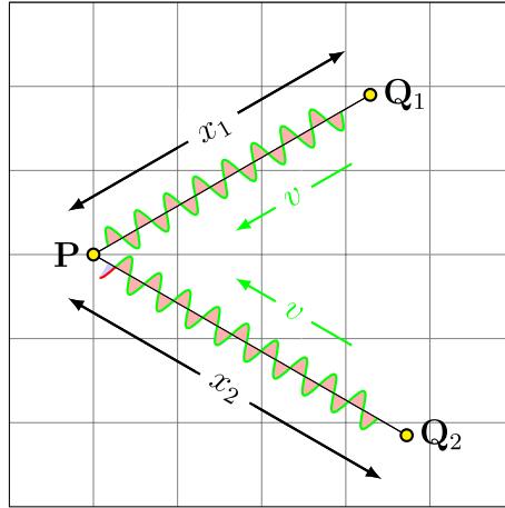
Abbildung 1.22: Gangunterschied.
