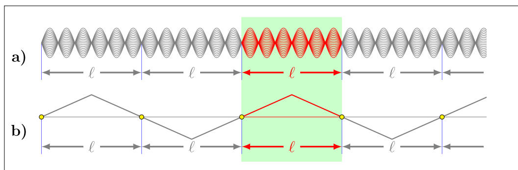
Abbildung 1.34: Durch das beidseitige Einspannen einer Saite bedingte periodische Randbedingungen: a) 6. Harmonische, b) gezupfte Saite
