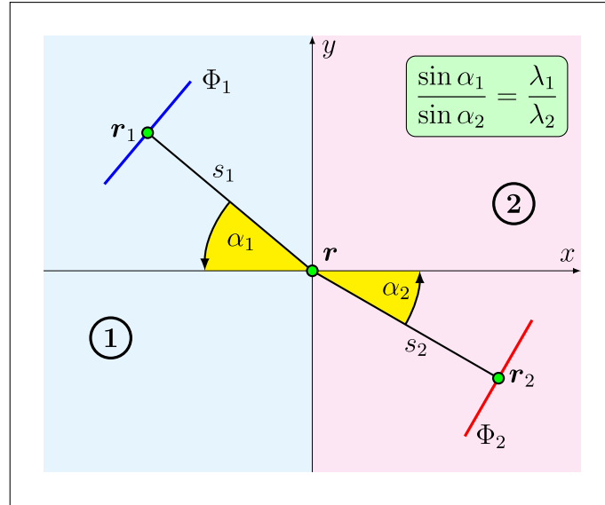
Abbildung 1.45: Fermat'sches Prinzip und Brechungsgesetz.
