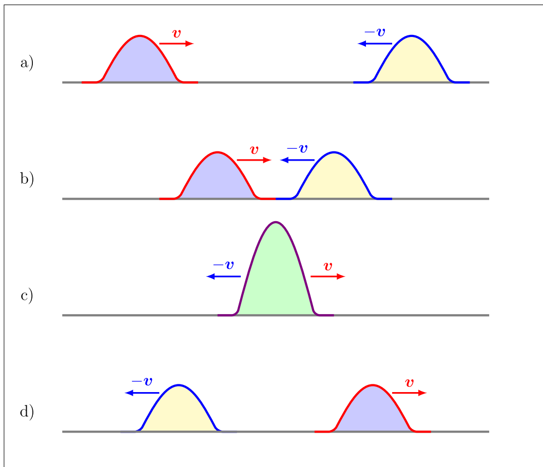
Abbildung 1.20: Zwei Wellen begegnen sich. In c) ist die resultierende Amplitude gleich der Summe der Amplituden der beiden einlaufenden Wellen.
