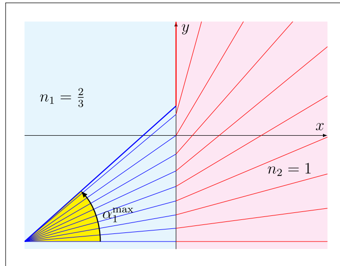
Abbildung 1.46: Brechung und Totalreflexion beim Übergang vom optisch dichteren zum optisch dünneren Medium.
