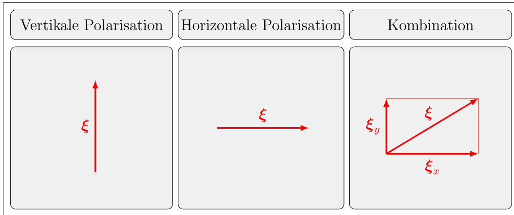
Abbildung 1.16: Lineare Polarisation.
