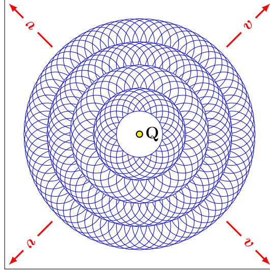
Abbildung 1.38: Huygens'sches Prinzip bei einer Kugelwelle (Quelle Q ).
