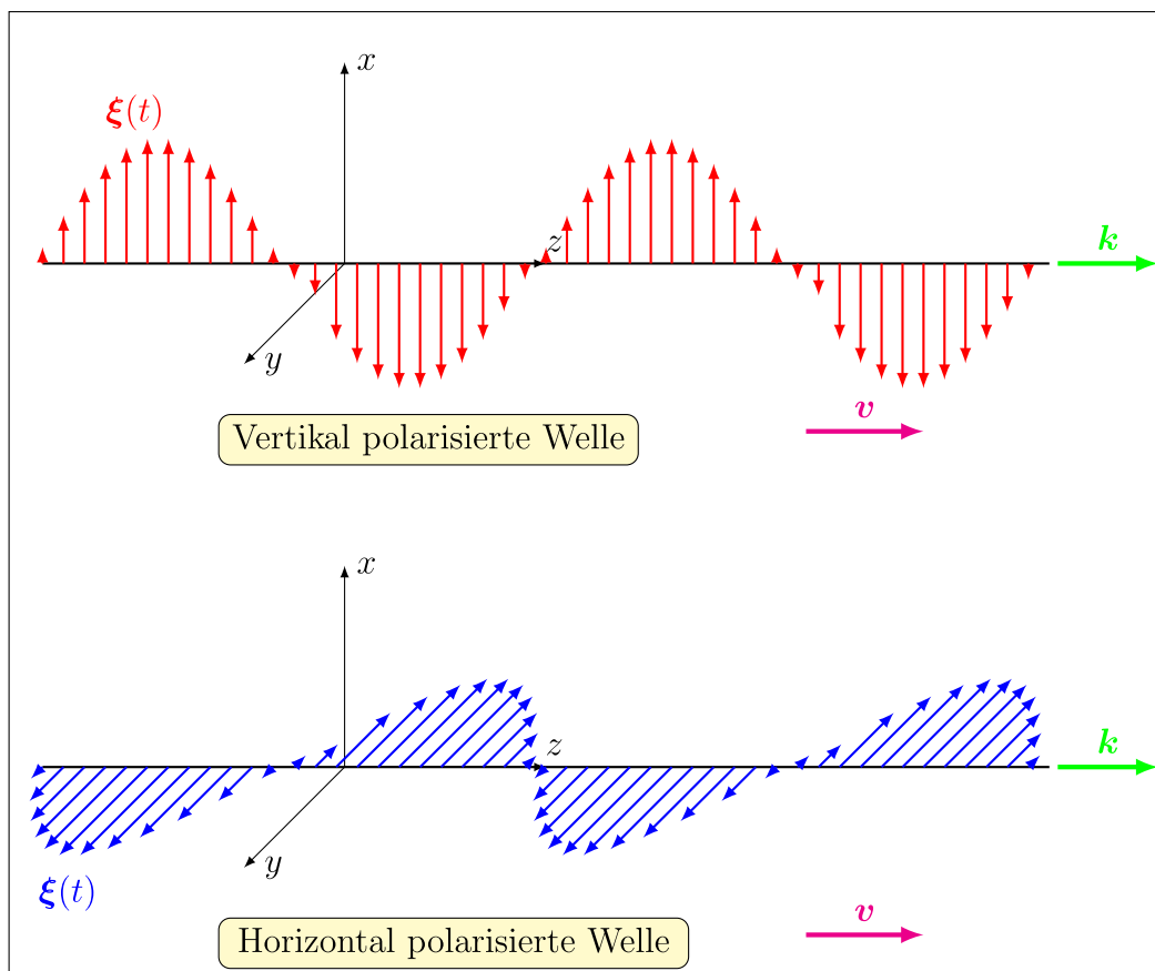
Abbildung 1.17: Horizontal bzw. vertikal polarisierte Welle.
