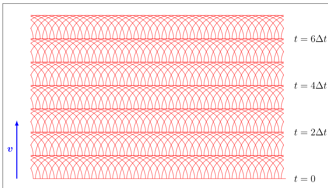
Abbildung 1.37: Huygens'sches Prinzip bei einer ebenen Wellenfront.
