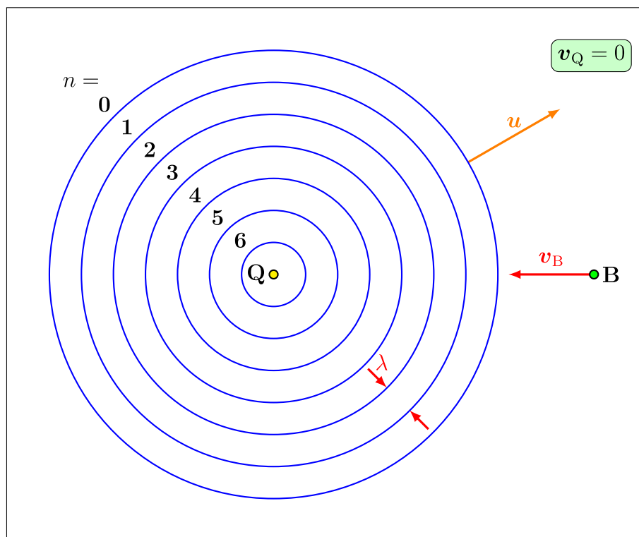
Abbildung 1.55: Dopplereffekt: Ruhende Quelle, bewegter Beobachter.
