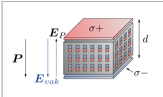
(b) Plattenkondensator mit Dielektrikum. Wir stellen uns das Dielektrikum aus vielen kleinen elementaren Dipolen aufgebaut vor. Die elementaren Dipolmomente addieren sich zur Polarisation \mathbf{P} .
