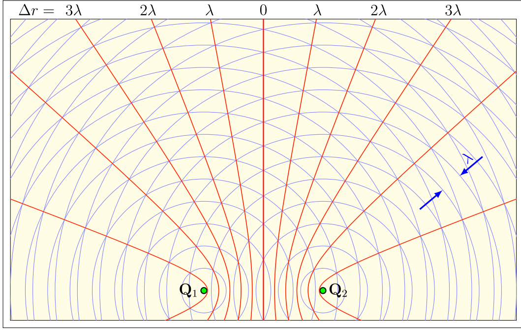
Abbildung 1.24: Interferenz zweier Kreiswellen mit fester Phasenbeziehung.
