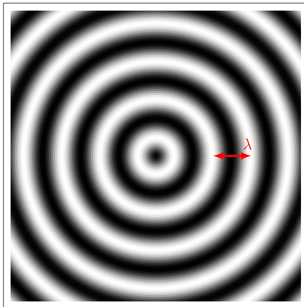
Abbildung 1.19: Longitudinale Kugelwellen.
