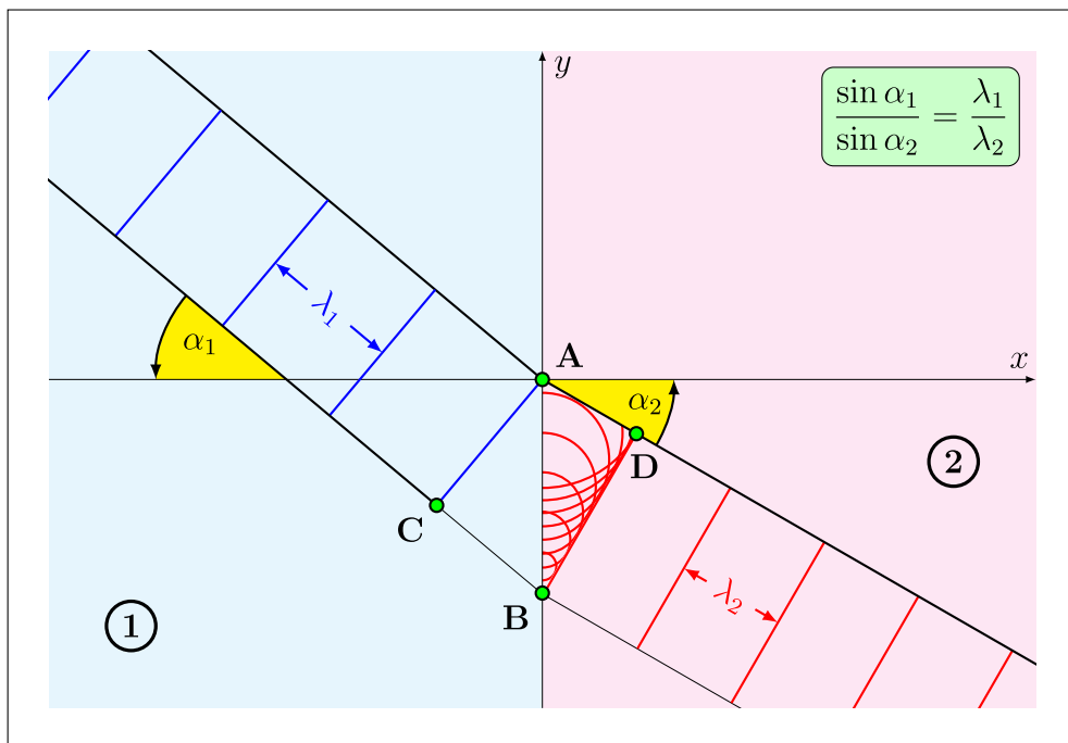
Abbildung 1.44: Huygens'sches Prinzip und Brechungsgesetz.
