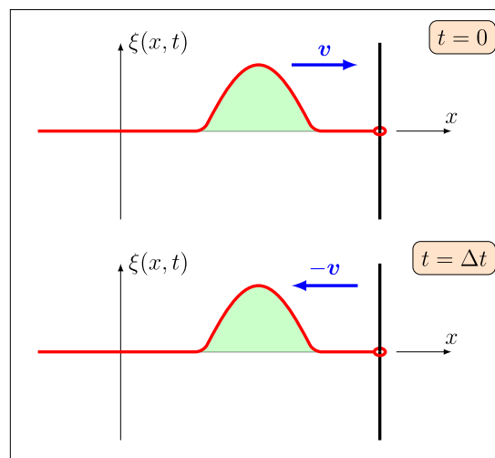
Abbildung 1.27: Reflexion eines Wellenberges am losen Ende.
