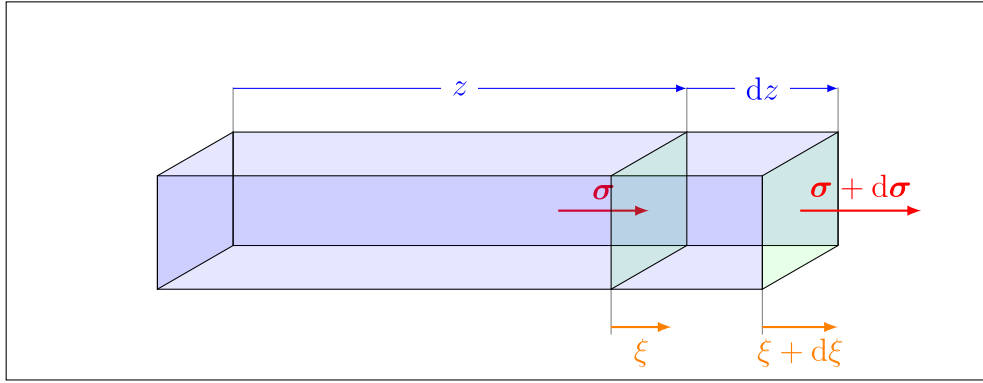
Abbildung 1.14: Zur Herleitung der Wellengleichung in einem Stab.
