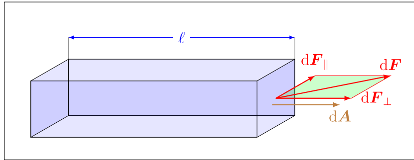
Abbildung 1.11: Zur Herleitung von Zug- und Schubspannung. Beachten Sie, dass im Bild das Flächenelement da mit dA bezeichnet ist.
