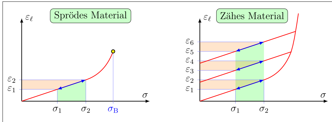
Abbildung 1.13: Plastische und elastische Verformung unter dem Einfluss einer Zugspannung \sigma . Sprödes Material bricht bei der Bruchspannung \sigma_b .
