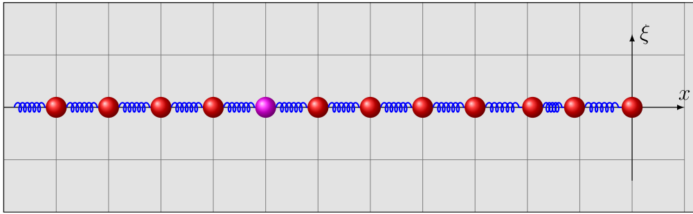
Abbildung 1.3: Longitudinale Wellen im Masse-Feder-System. Die zweite und dritte Masse von rechts sind aus ihrer Ruhelage ausgelenkt.
